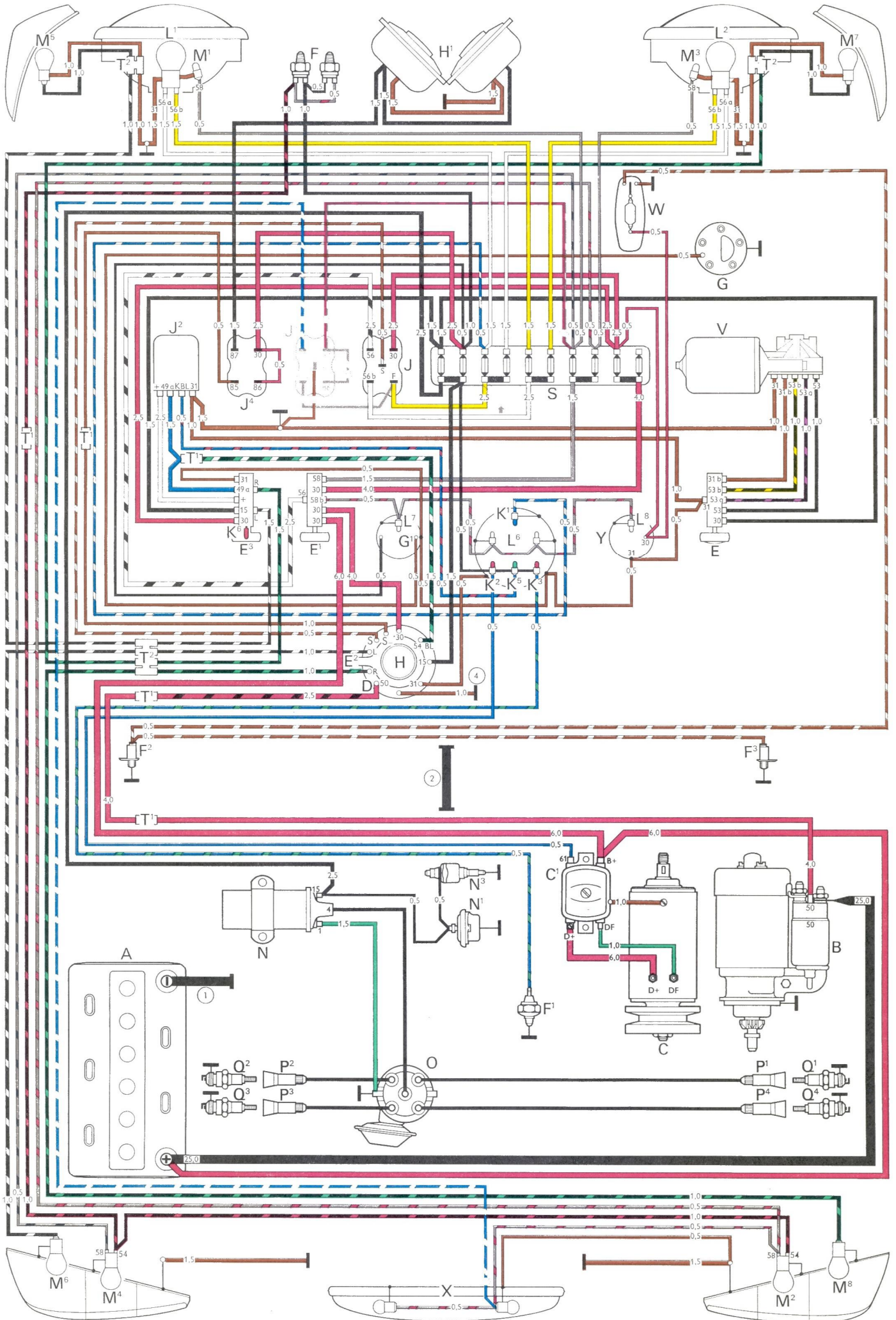
Schaltplan VW 1500 Karmann Ghia ab August 1969
